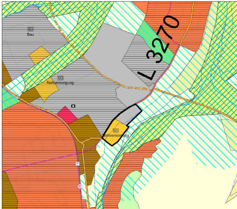
Abbildung 3: Ausschnitt aus dem Regionalen Flächennutzungsplan des Regionalverbandes Frankfurt/ Rhein-Main (Stand Juni 2020). Das Plangebiet ist schwarz markiert.
