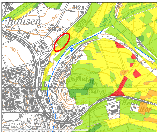
Abbildung 9: Bodenfunktionsbewertung im Plangebiet und seiner Umgebung. Hellgrün dargestellt sind Flächen geringer Bedeutung (Stufe 2 von 5), gelb sind Flächen mit mittlerer Bedeutung (Stufe 3 von 5). Das Plangebiet ist rot markiert.
