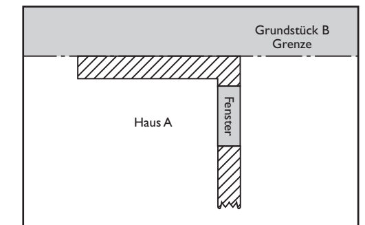
Außenwand stößt senkrecht auf Grundstücksgrenze: Fenster ohne Einhaltung eines Abstandes zulässig.
