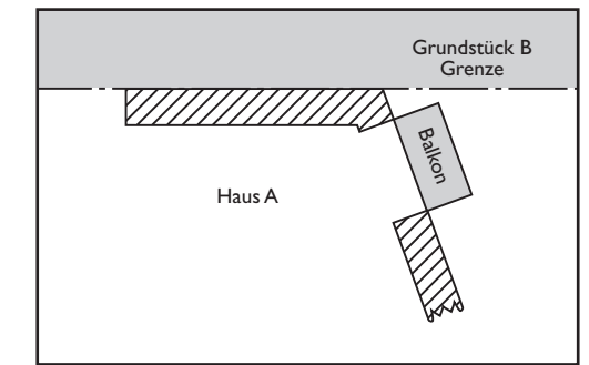
Außenwand verläuft im Winkel von 70 Grad zur Grundstücksgrenze: Balkon ohne Einhaltung eines Abstandes zulässig.
