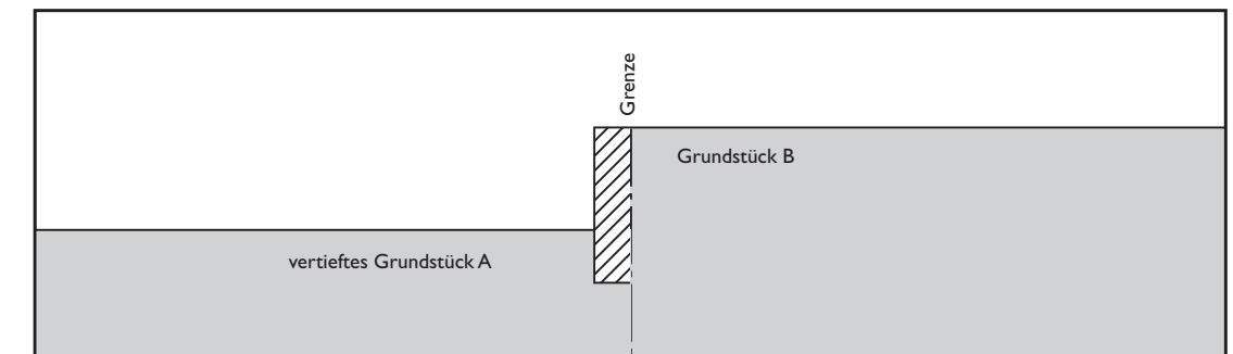
Zulässige Vertiefung mit Stützmauer
